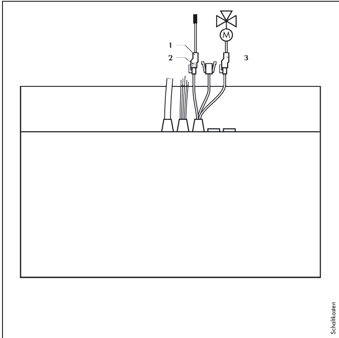
Рис. 5.3 Электрическое подключение
