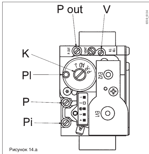
газовый клапан SIT модели SIGMA 848
