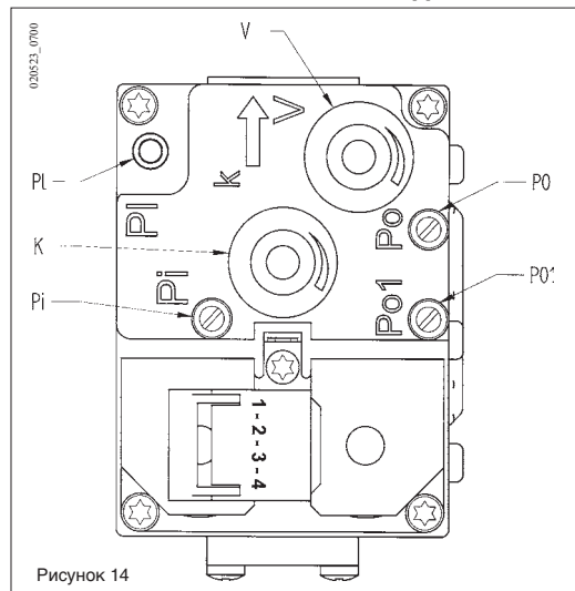
газовый клапан SIEMENS модели VDU 11
