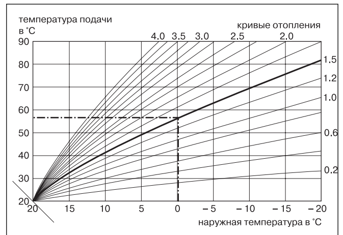
Рис. 4.15 Диаграмма с кривыми отопления для заданной комнатной температуры 20 °C
