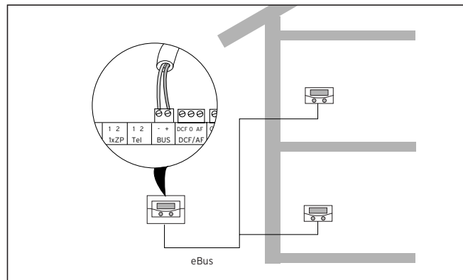
Рис. 4.8: Подключение устройств дистанционного управления
