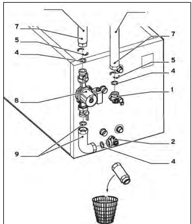
Рис . 7: Монтаж присоединительного комплекта водонагревателя на uniSTOR VIH H 120 - 200
