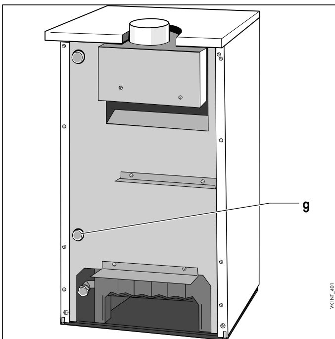
Рис.4.1 Подключение к газопроводу
