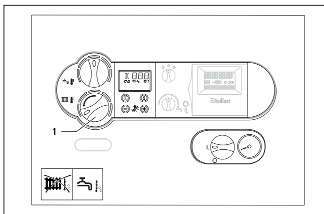
Рис. 4.8 Отключение режима отопления (летний режим)
