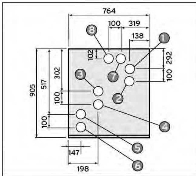
Рис. 5.2 Подсоединения и размеры
