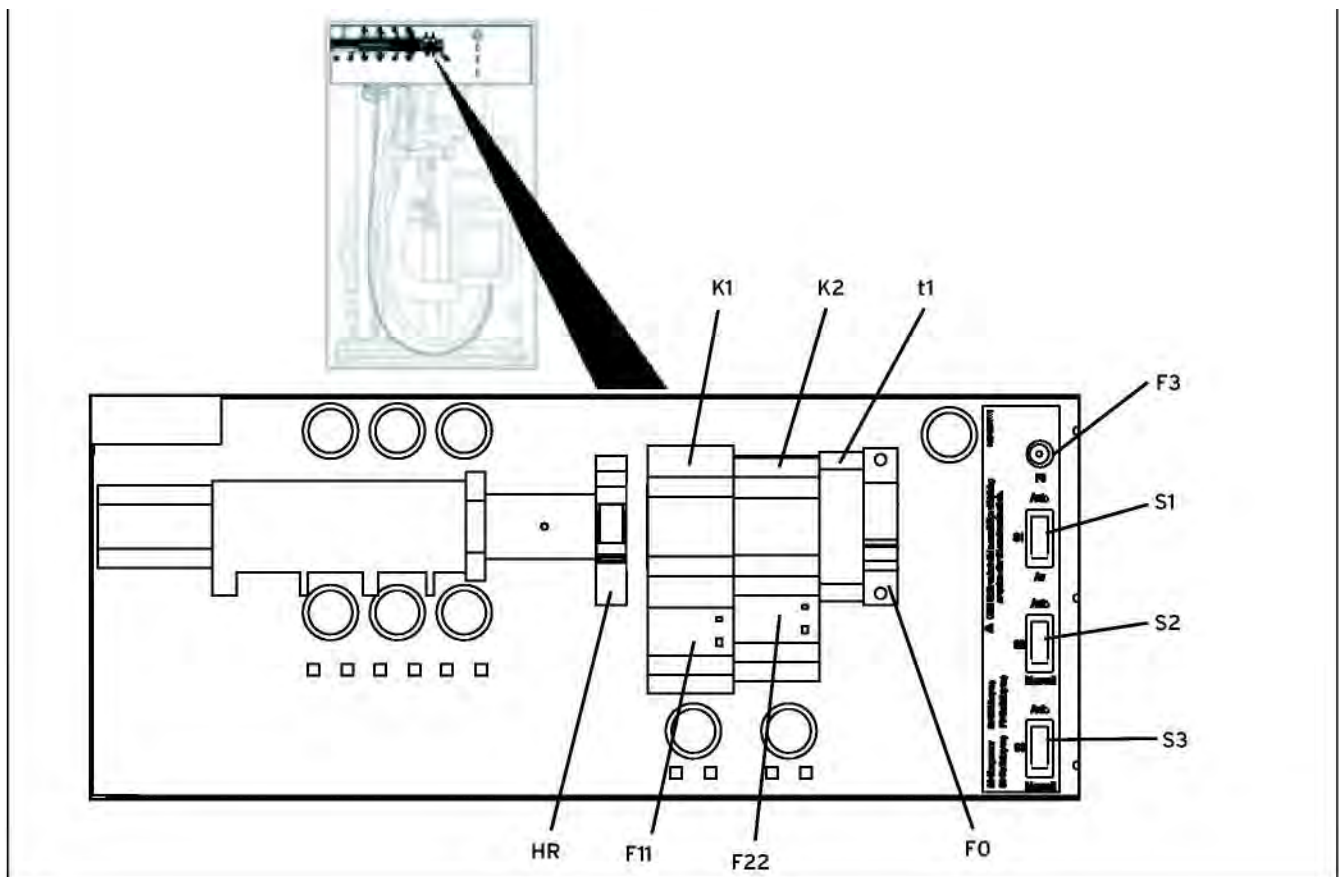
Рис. 7.4 Местоположение защитных предохранителей
