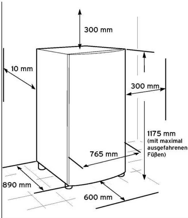
Рис. 3.5 Требуемое свободное монтажное пространство
