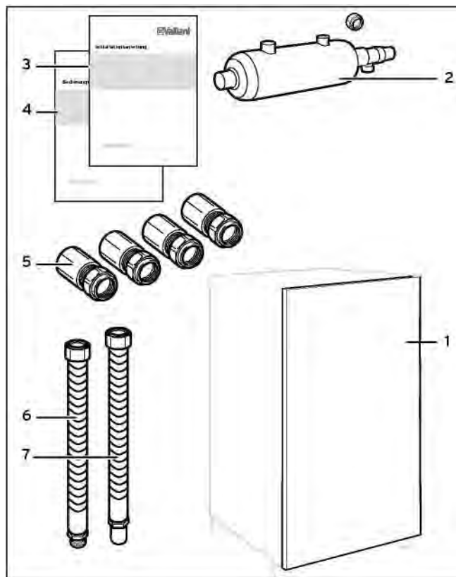
Рис. 3.3 Объем поставки
