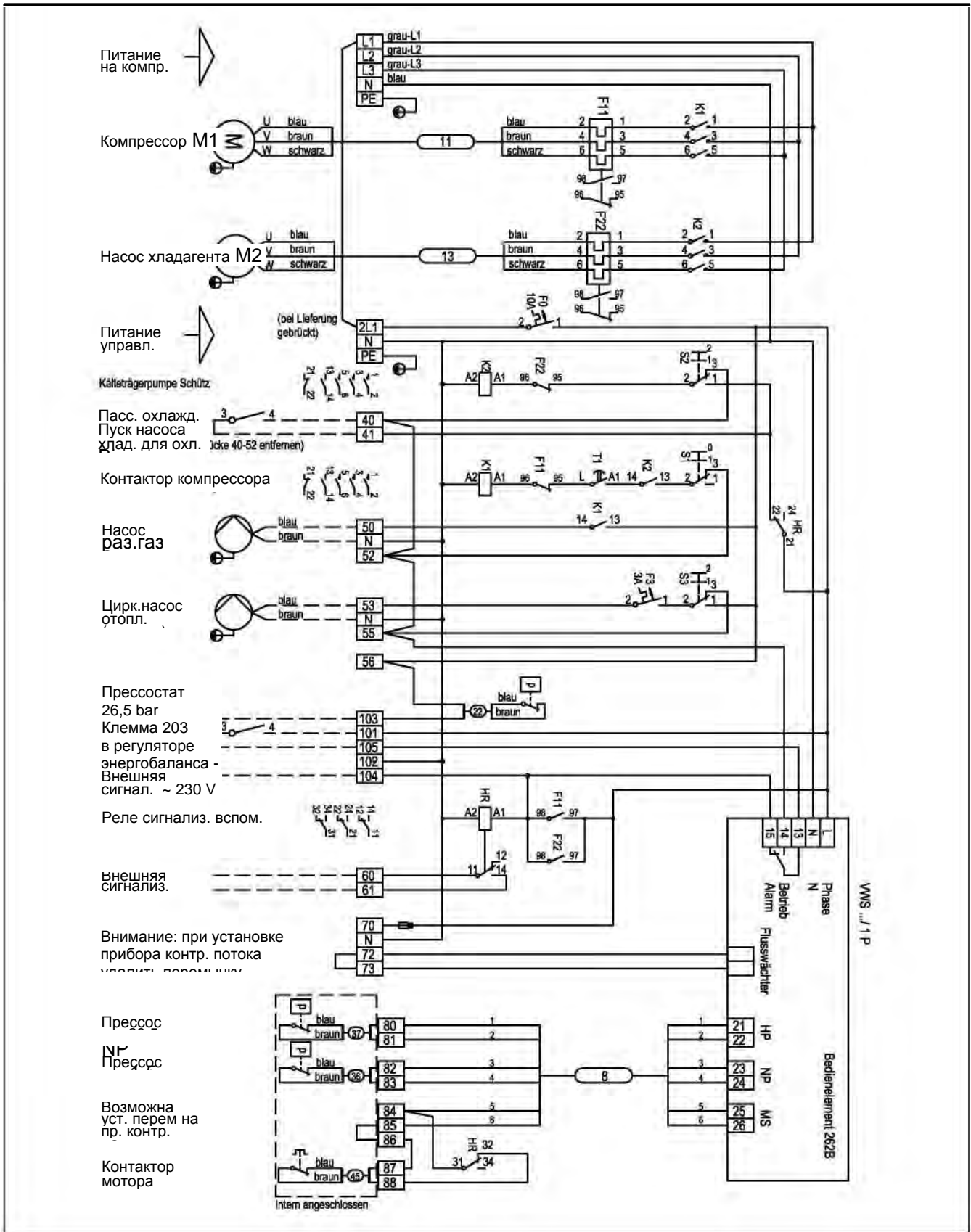
Рис. 7.5 Коммутационная схема VWS 22/1, 28/1, 38/1, 44/1 P
