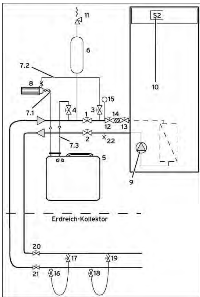
Рис. 7.2 Наполнение циркуляционного контура хладагента
