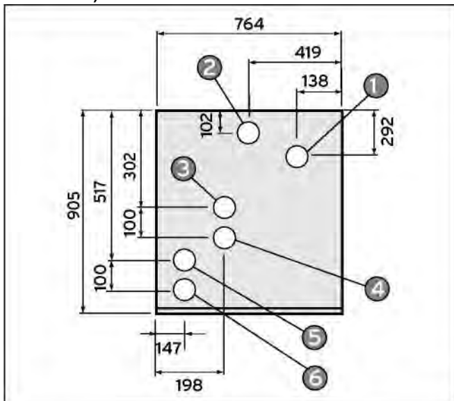
Рис. 5.1 Подсоединения и размеры
