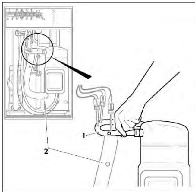
Рис. 9.1 Проверка направления вращения компрессора и изменение направления при необходимости
