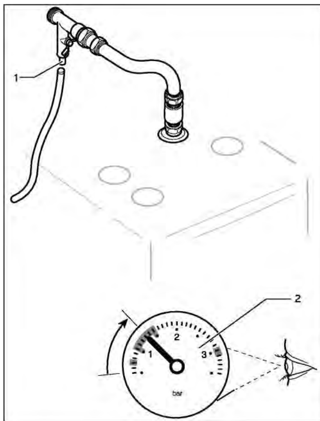
Рис. 6.1 Наполнение системы отопления
