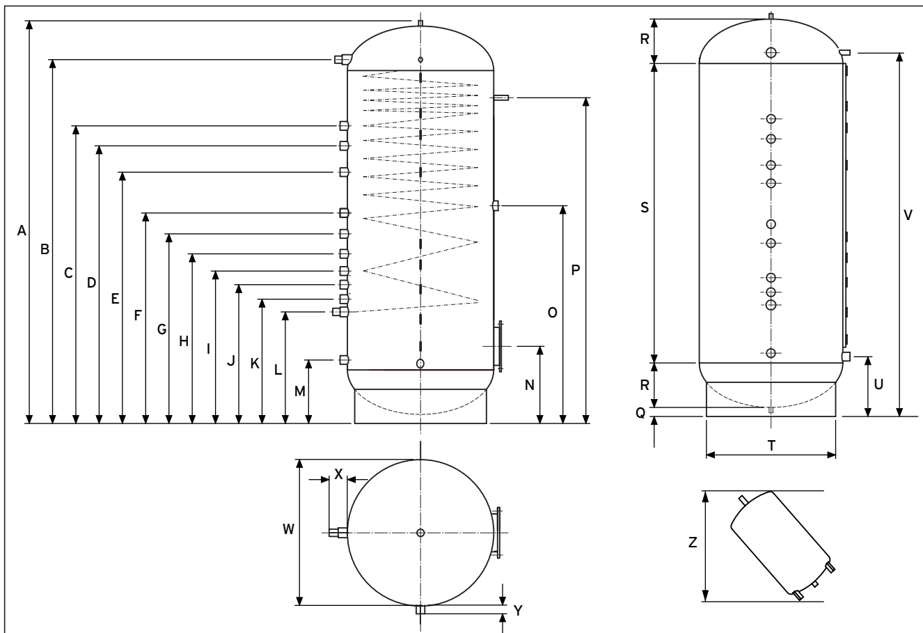
Рис. 4.3 Размеры
