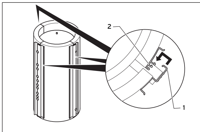
Рис. 4.6 Фиксация зажимных планок
