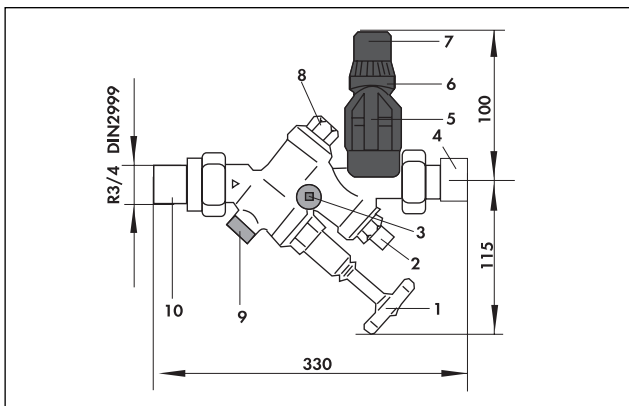
Рис.1 Элементы группы безопасности
