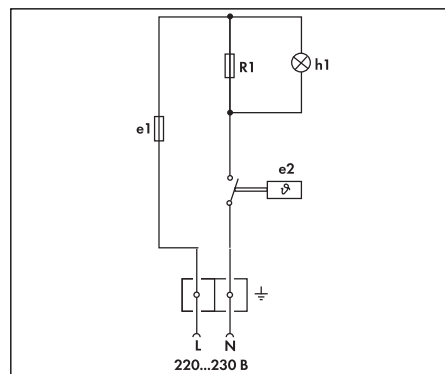
Рис. 8 Электрическая схема
