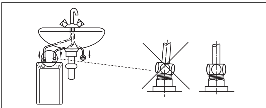
Рис. 7 Подсоединение арматуры без перекосов
