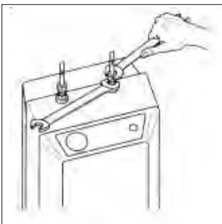
Рис. 6 Способ подсоединения арматуры
