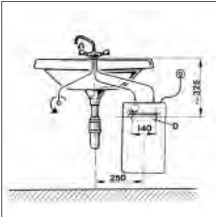
Рис. 3 Пример монтажа, Размеры в мм
