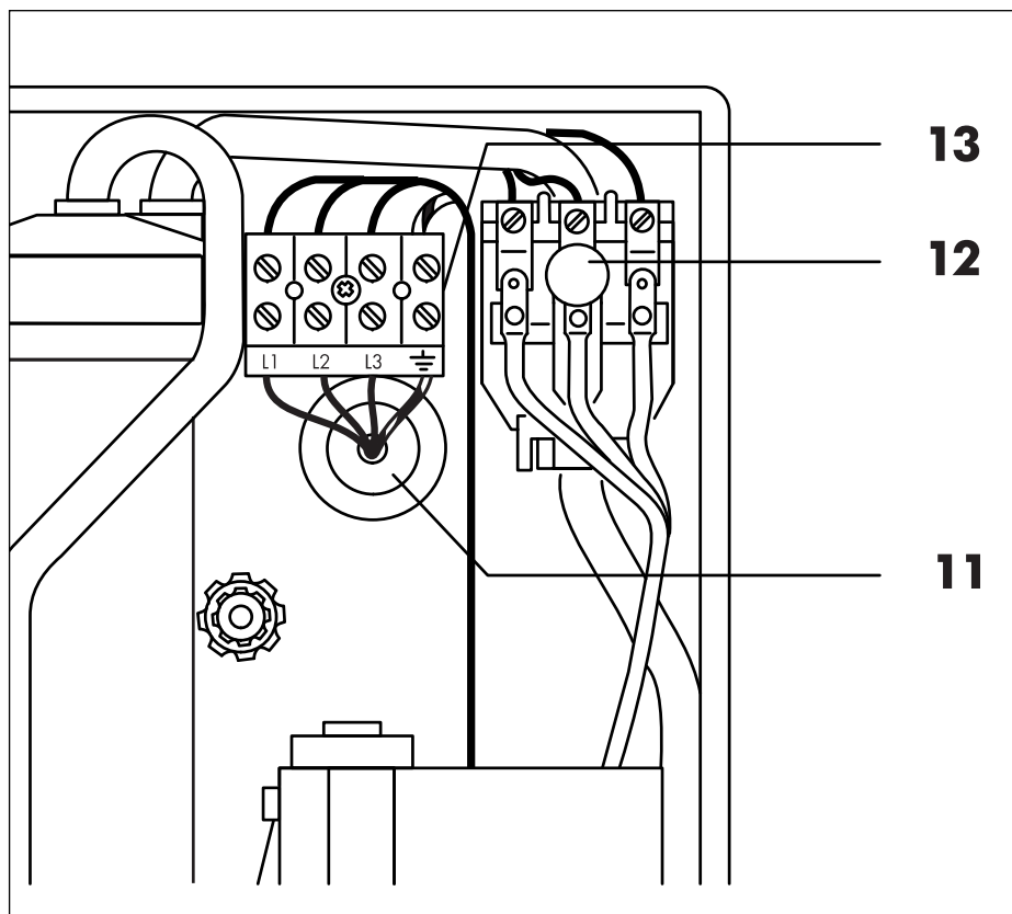
Рис. 6.1 Ввод электрического кабеля в верхней части прибора
