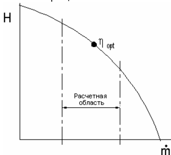
Характеристическая кривая циркуляционного насоса
