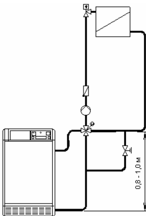
Основная схема включения четырехходового смесителя
