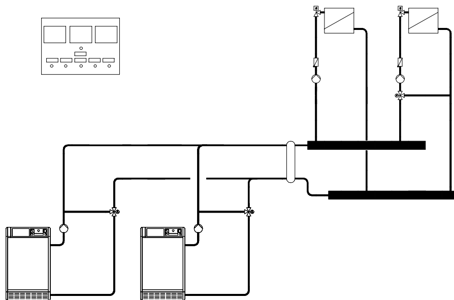
Регулируемое повышение температуры обратной воды
