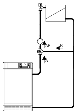
Регулирование смеси (правое подключение)
